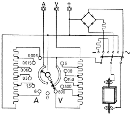
Schaltbild 2
